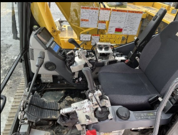
バックホウ無人運転席
